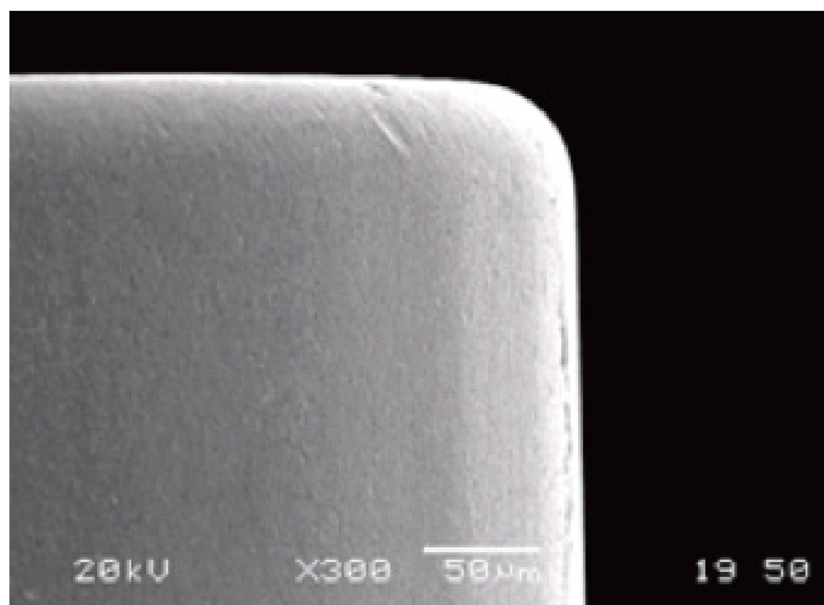
図1 端部R加工例
